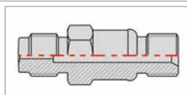
Raccordo entrata
