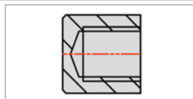
Raccordo premimolla 02-
